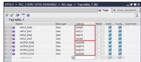
Figura 103 – Tabela de tags do CLP
