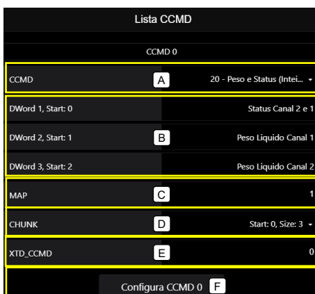
Figura 35 – Informação da terminação da porta serial
