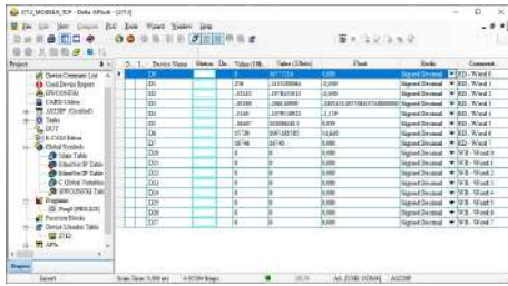
Figura 127 – Dados da comunicação Modbus TCP
