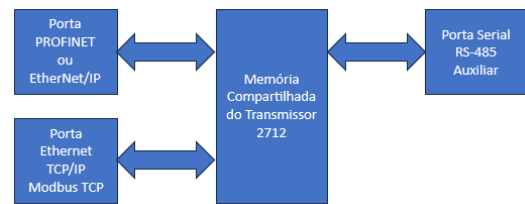
Figura 141 – Exemplo das conexões possíveis
