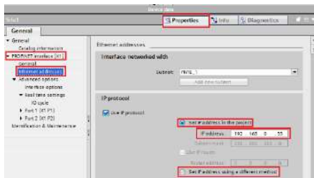
Figura 99 – Propriedades do Transmissor → configuração IP
