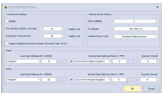
Figura 122 – Configurações da comunicação Modbus TCP
