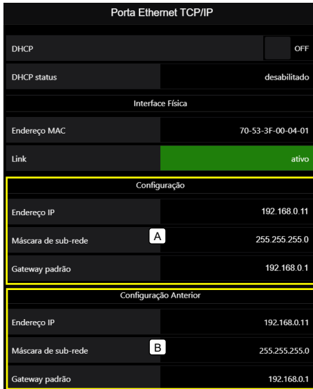
Figura 9 – Transmissor de Pesagem Automática 2712 em modo RESET IP (carrega as configurações de fábrica)
