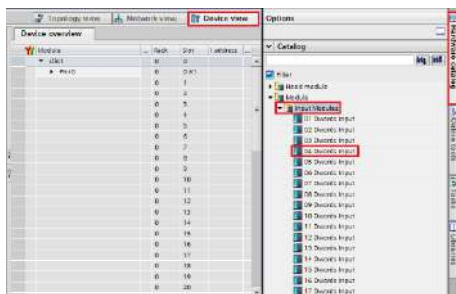
Figura 100 – Mapeamento da área de dados
