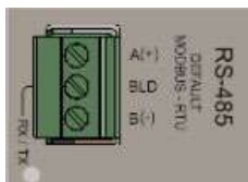
Figura 129 – Porta Modbus RTU
