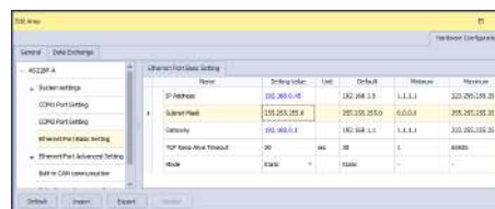
Figura 119 – Configurações Ethernet do controlador
