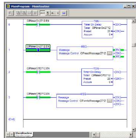
Figura 73 – Estrutura do programa no RSLogix 5000
