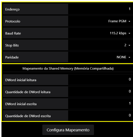
Figura 128 – Tela de configuração dos parâmetros do Modbus RTU
