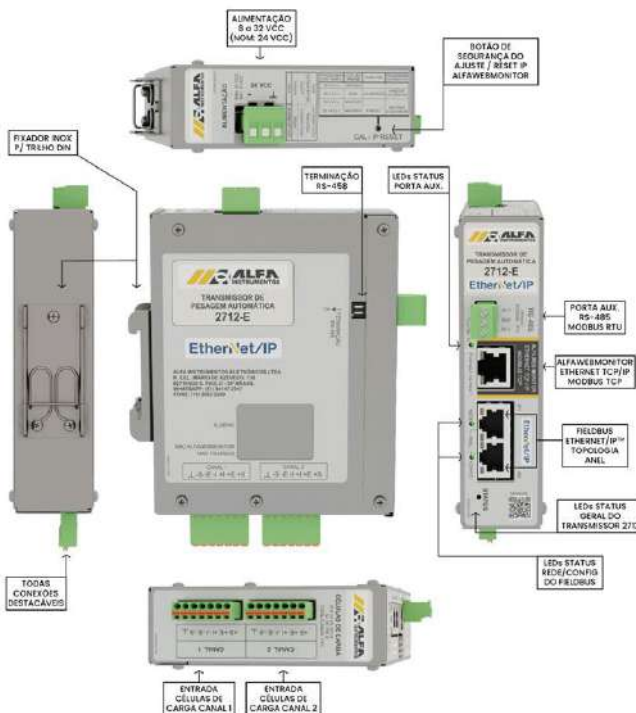
Figura 1 – Transmissor de Pesagem Automática 2712
