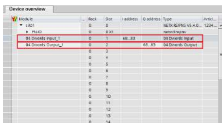
Figura 101 – Endereçamento dos tags do Transmissor
