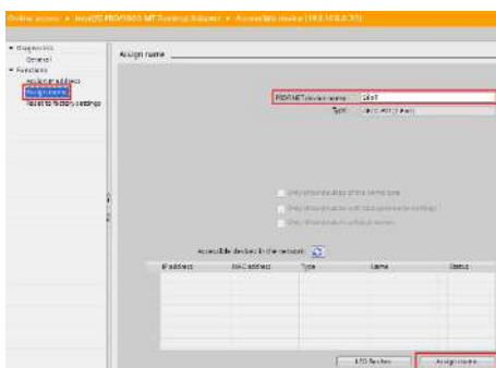
Figura 91 – Configuração do PROFINET device name
