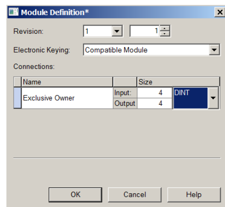
Figura 64 – Tela de configuração de DWs de Input e Output
