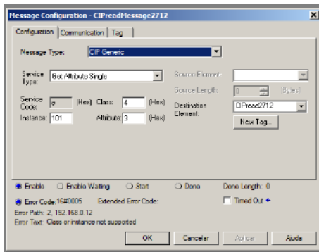
Figura 77 – Configuração Read Message para RSLogix 5000
