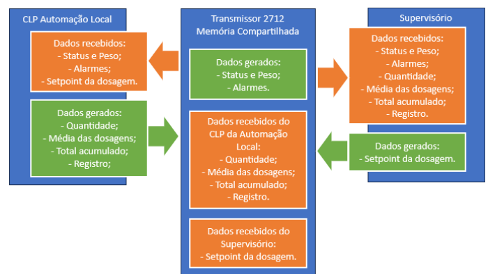
Figura 142 – Exemplo da troca de dados entre as portas de comunicação utilizando a Memória Compartilhada do Transmissor 2712
