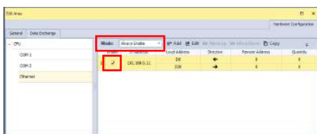
Figura 123 – Habilitação da comunicação Modbus TCP
