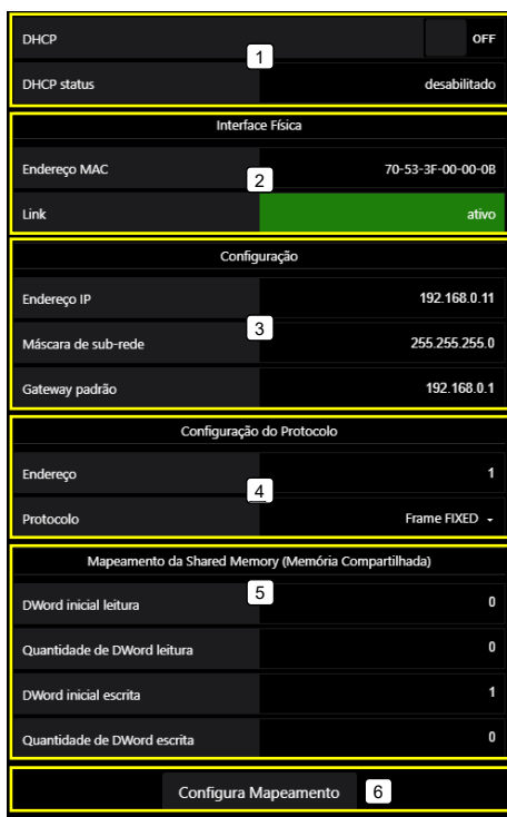
Figura 115 – Tela de configuração dos parâmetros Ethernet TCP/IP
