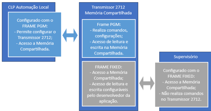
Figura 143 – Exemplo de uso das portas de comunicação com a Memória Compartilhada.
