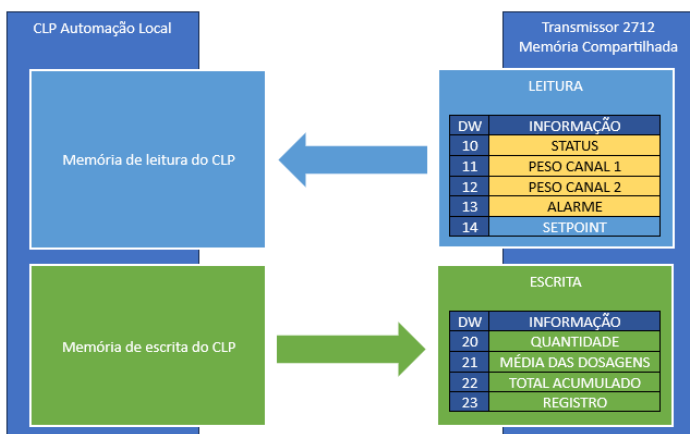
Figura 144 – Exemplo da troca de dados do CLP configurado com PGM e acesso a Memória Compartilhada
