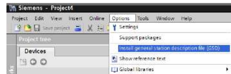
Figura 86 – Instalação arquivo GSDML
