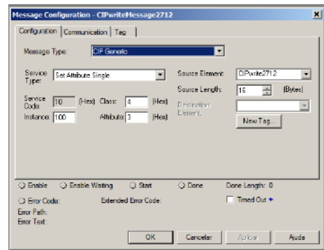
Figura 81 – Configuração Write Message para RSLogix 5000
