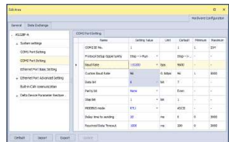
Figura 132 – Configurações Modbus RTU do controlador
