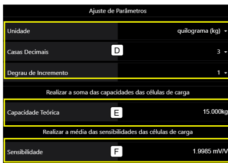
Figura 46 – Tela de Ajuste do Canal
