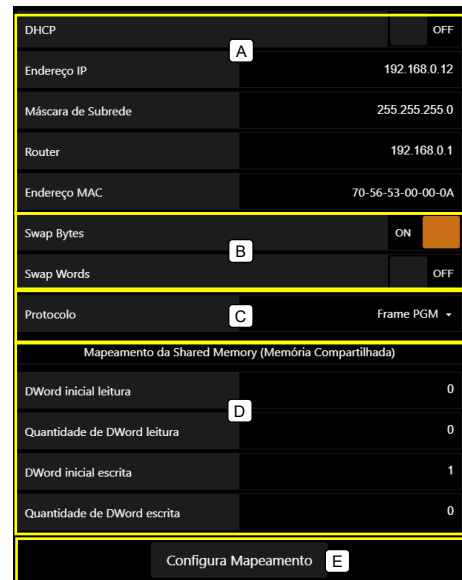
Figura 56 – Tela de configuração dos parâmetros EtherNet/IP™
