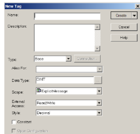
Figura 74 – Janela New Tag RSLogix 5000
