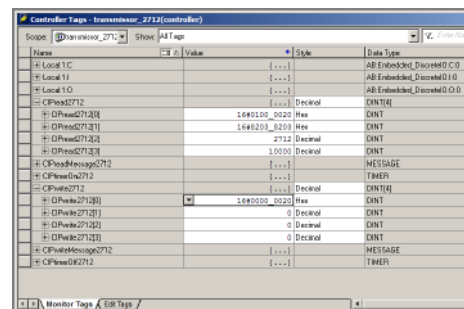
Figura 83 – Controler Tags RSLogix 5000
