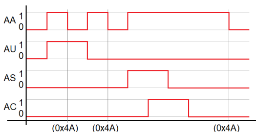
Figura 153 – Comportamento do acionamento do bit AA (Alteração do Alarme)
